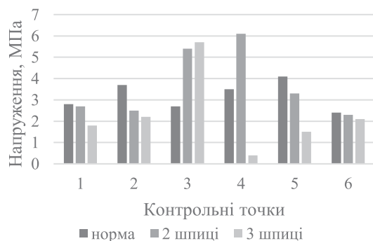
Рис. 7. Діаграми величин напруження в контрольних точках моделей плечової кістки з косим надвиростковим переломом під впливом розтягувального навантаження: а – у кісткових елементах; б – у шпицях
