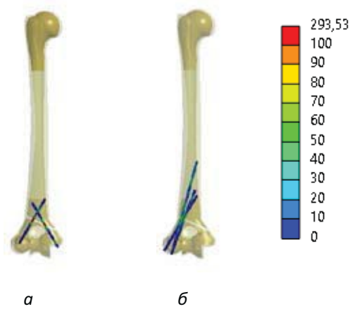
Рис. 9. Розподіл напруження в шпильках моделей плечової кістки під впливом навантаження на згинання: а – перехресна фіксація 2 шпильками; б – латеральна фіксація 3 шпильками
