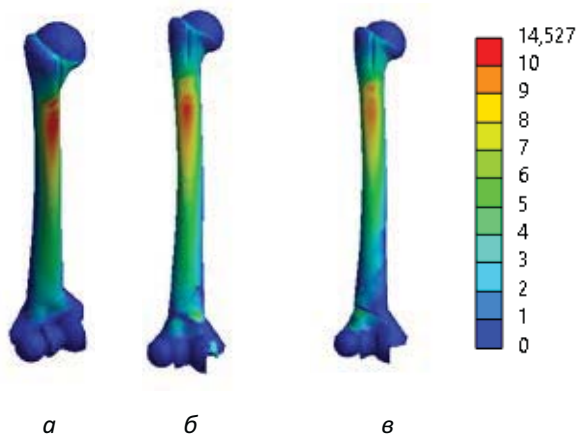
Рис. 8. Розподіл напруження в кісткових елементах моделей плечової кістки під впливом навантаження на згинання: а – у нормі; б – з косим переломом із перехресною фіксацією 2 шпильками; в – з косим переломом із латеральною фіксацією 3 шпильками
